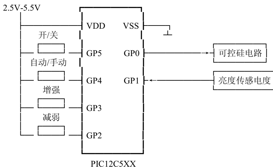
图 3.1 灯光调节器
