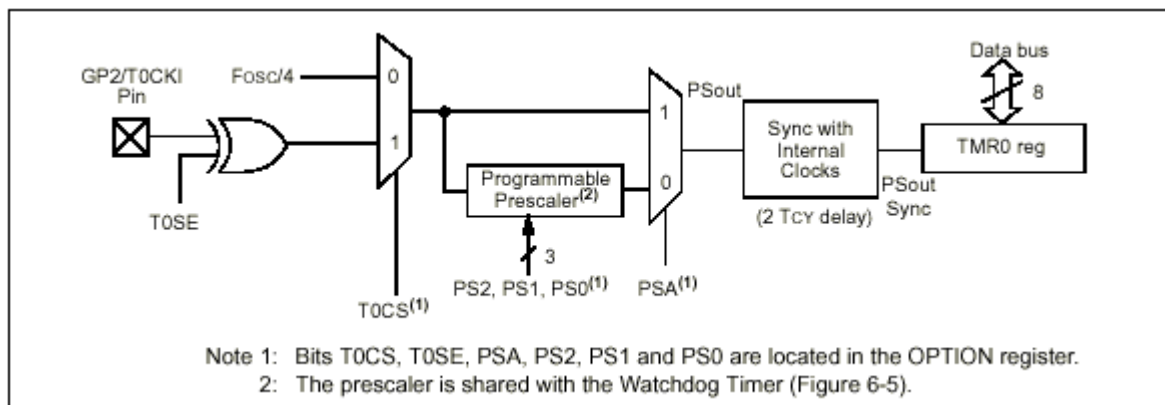
图 1.14 TIMER0 方块图
